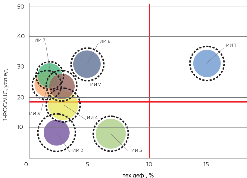
Рисунок 4 — Матрица по направлению компьютерная томография органов грудной клетки, целевая патология COVID-19. По горизонтальной оси — процент технологических дефектов (тех.деф.,%); по вертикальной оси — величина «1-ROCAUC».
